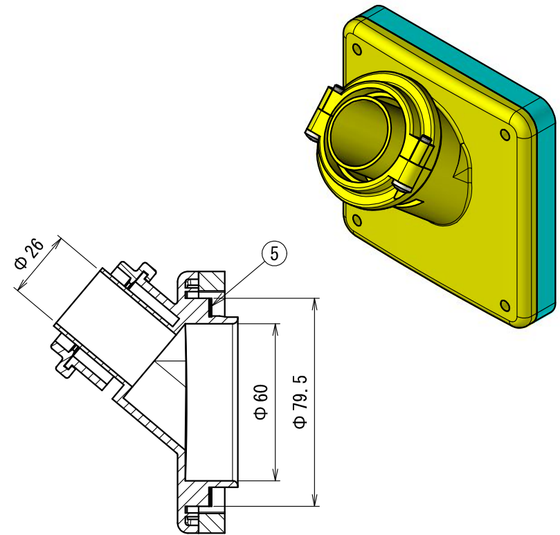
断面 A-A
